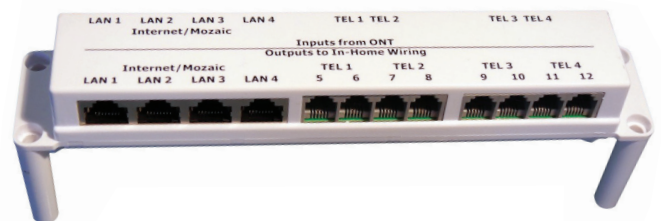
Optional Cat6 Patching Module
